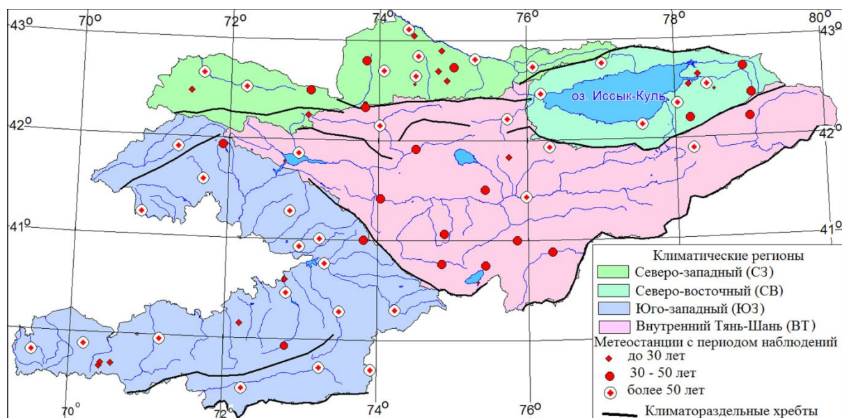
Рисунок. 2.1. Климатическое зонирование Кыргызской Республики и локализация метеостанций
