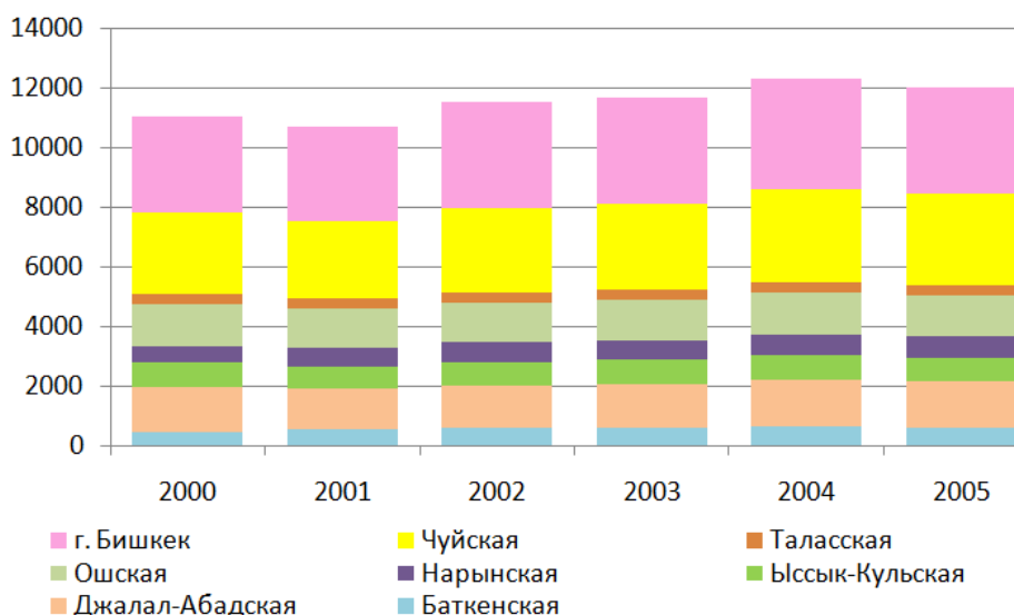
Рисунок 2.10. Распределение выбросов по административным единицам, тыс. т CO 2 -экв
