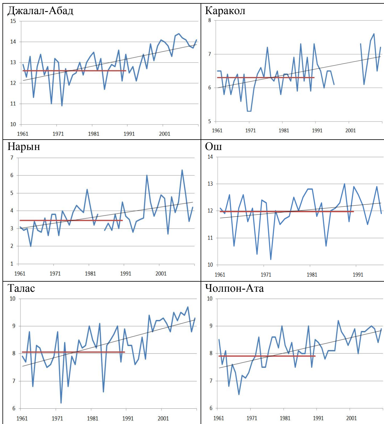
Рисунок 2.5. Тенденции изменения среднегодовой температуры относительно базового периода (1961 – 1990 гг.).
