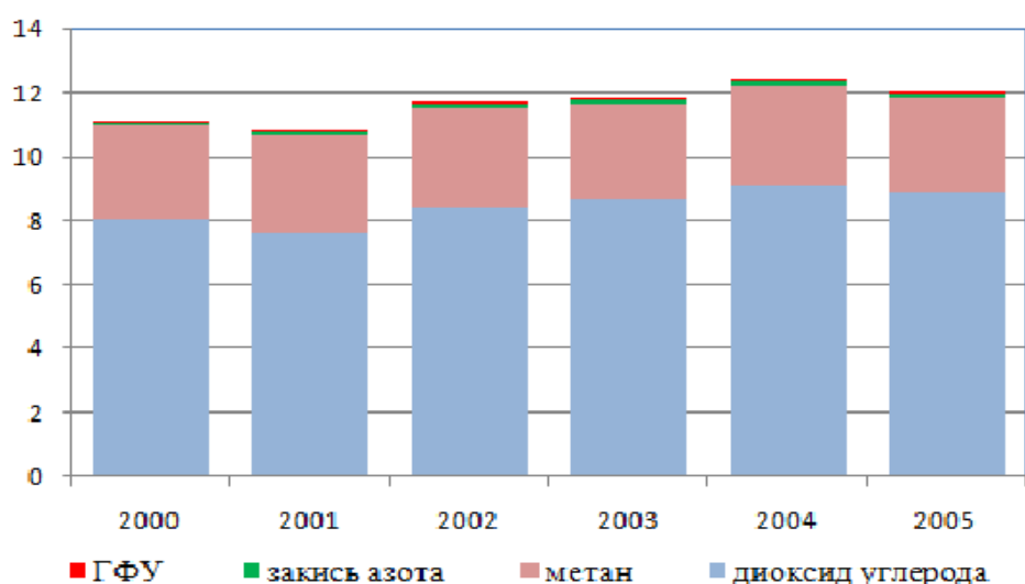
Рисунок 2.9. Выбросы основных парниковых газов, млн. т CO 2 -экв.
