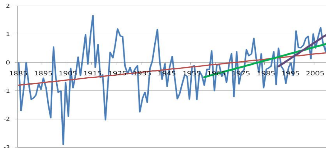
Рисунок. 2.3. Тенденции изменения среднегодовых значений приземной температуры во времени. В скобках показана скорость изменения температуры для отдельных временных периодов в °С/100 лет
