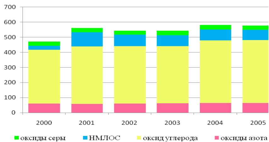
Рисунок 2.12. Эмиссия прекурсоров по газам, метрических тыс. тонн
