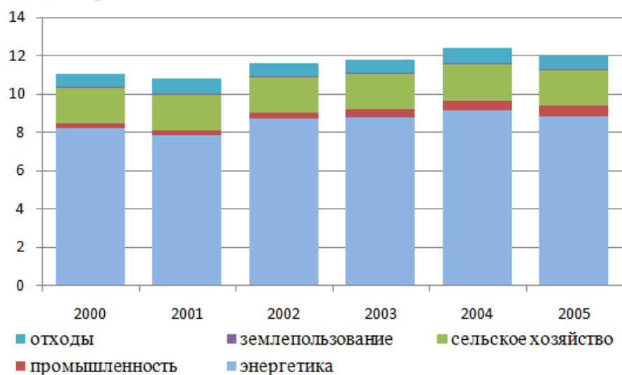
Рисунок 2.8. Динамика выбросов парниковых газов по основным секторам (без учета стоков), млн. т CO 2 -экв.
